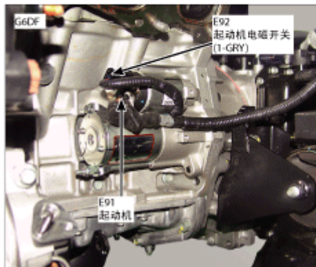
193.发动机左侧
