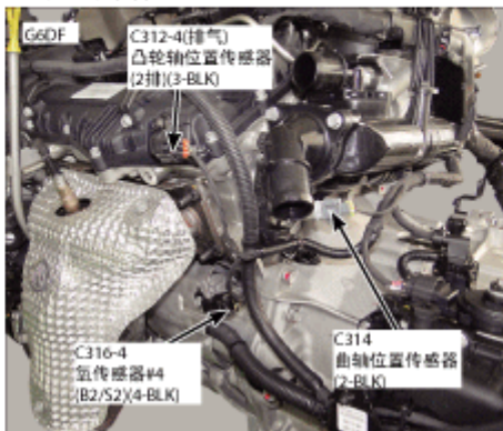
194.发动机后部
