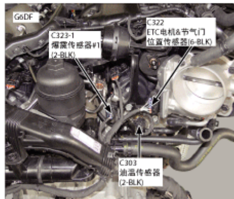
195.发动机后部
