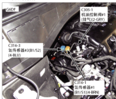
198.发动机前部
